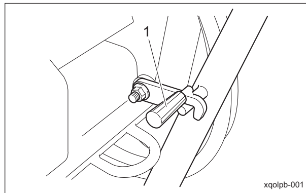
モアロックレバー（ラッチ）_001
