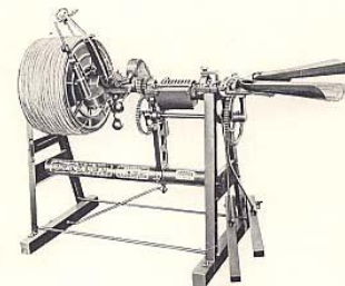
全鋼制馬沙尔式制縄机
